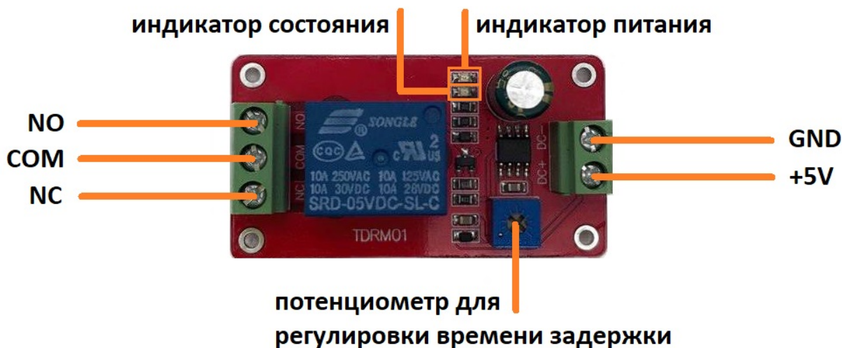
Рис. 1. Схема подключения реле с задержкой TDRM01-5V
