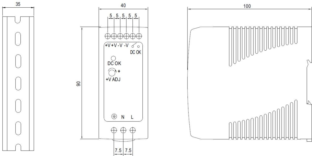
Рис. 1. Габариты источников питания MDR-40
