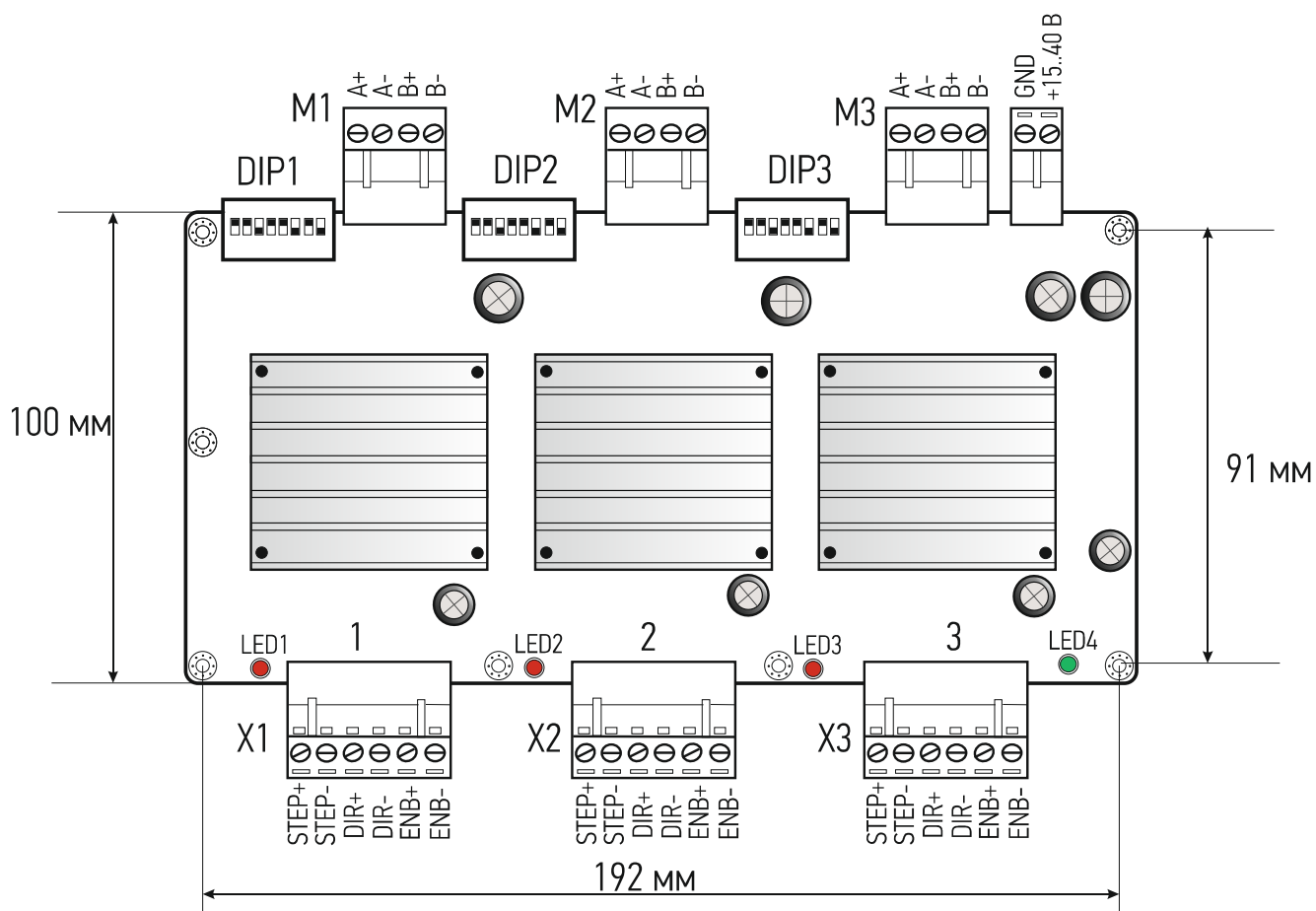
Рис. 1 Размеры устройства и основные разъемы
